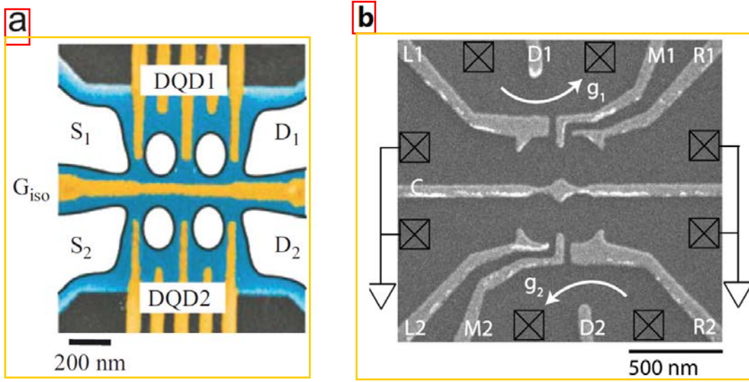
图 4.1 不同双电荷量子比特设计结构。(a) Fujisawa 小组设计的双电荷量子比特的 SEM 图片。(b) Ritchie 小组设计的双电荷量子比特的 SEM 图片。图片引自文献[2,5]。
