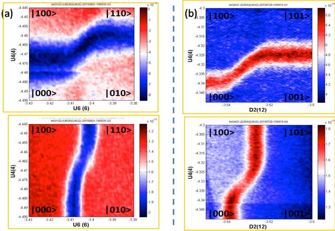
图 5.5 量子比特之间耦合能量 J 的测量。(a)量子比特 1 与 2 之间耦合能量 J_{12} 的测量图像,测量结果 J_{12}=95\text{ueV} 。(b)量子比特 1 与 3 之间耦合能量 J_{13} 的测量图像,测量结果 J_{13}=140\text{ueV} 。
