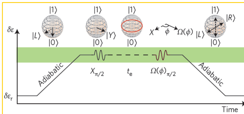
图 3.8 Ramsey 操作波形示意图。图片引自文献[12]。
