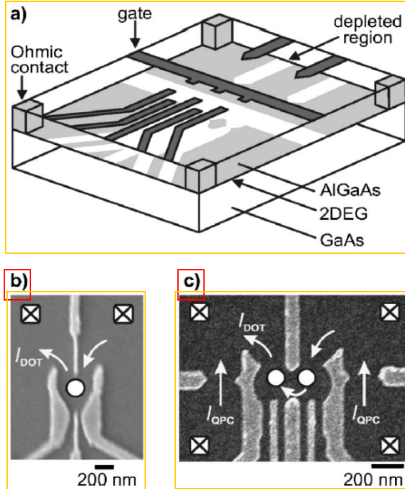
图 1.3 (a) 横向量子点结构示意图。在有二维电子气的 GaAs 通过表面栅电极上施加电压来排挤下面电子，将中间电子约束。(b)-(c) 扫描电子显微镜下单量子点和串联双量子点结构。(c)中两侧为量子点接触结构(QPC)。图片引自文献[31]。
