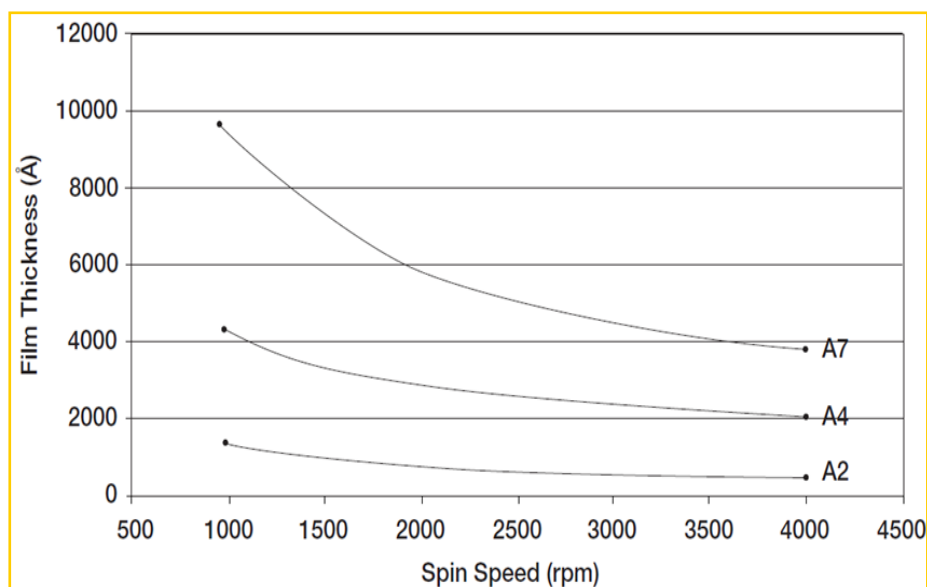
图 2.5 950PMMA 光刻胶匀胶转速与胶厚关系图。
