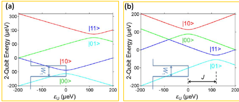
图 4.6 双电荷量子比特中计算的能级结构。(a)下面量子比特处于 |0\rangle_L 态时,上面量子点的平衡点在 \epsilon_U = 0 处。(b)下面量子比特处于 |1\rangle_L 态时,上面量子点的平衡点在 \epsilon_U = J 处。可以看到下面量子点的状态对上面量子点的平衡点的影响程度为 J 。图片引自文献[10]
