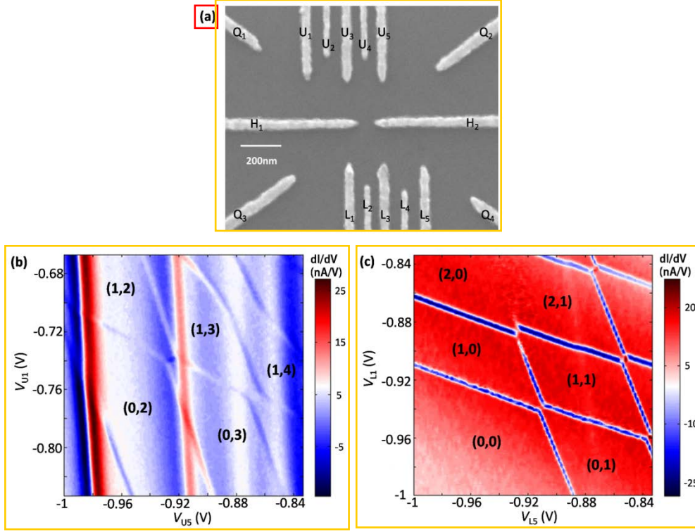
图 4.2 (a)我们的两电荷量子点样品 SEM 结构图。(b)和(c)分别为上面和下面双量子点的蜂窝图，(M,N)代表每个量子点中电荷的填充数目。图片引自文献[9]
