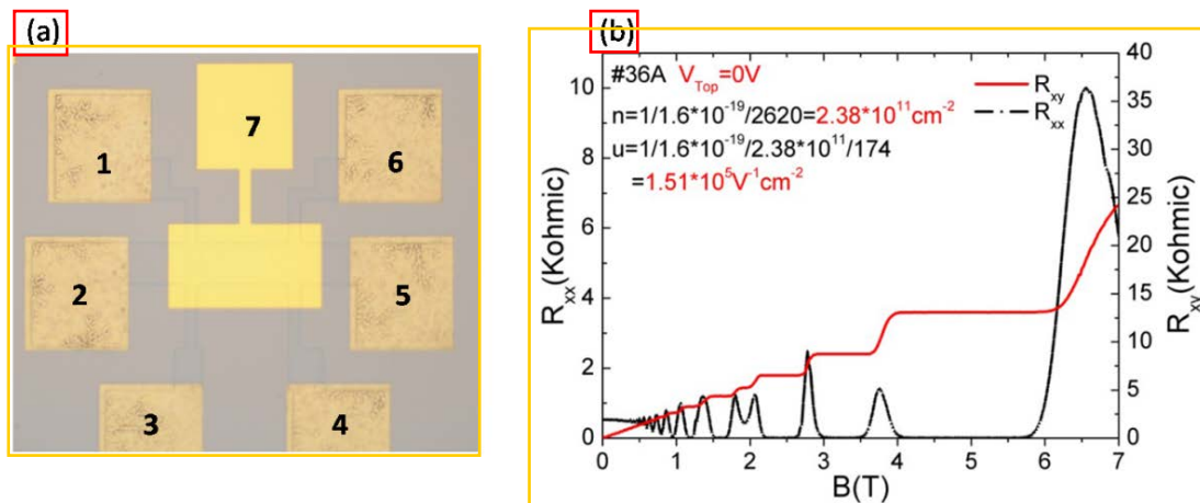
图 2.15 (a)Hall Bar 样品结构图。(b)测量的量子霍尔效应图。
